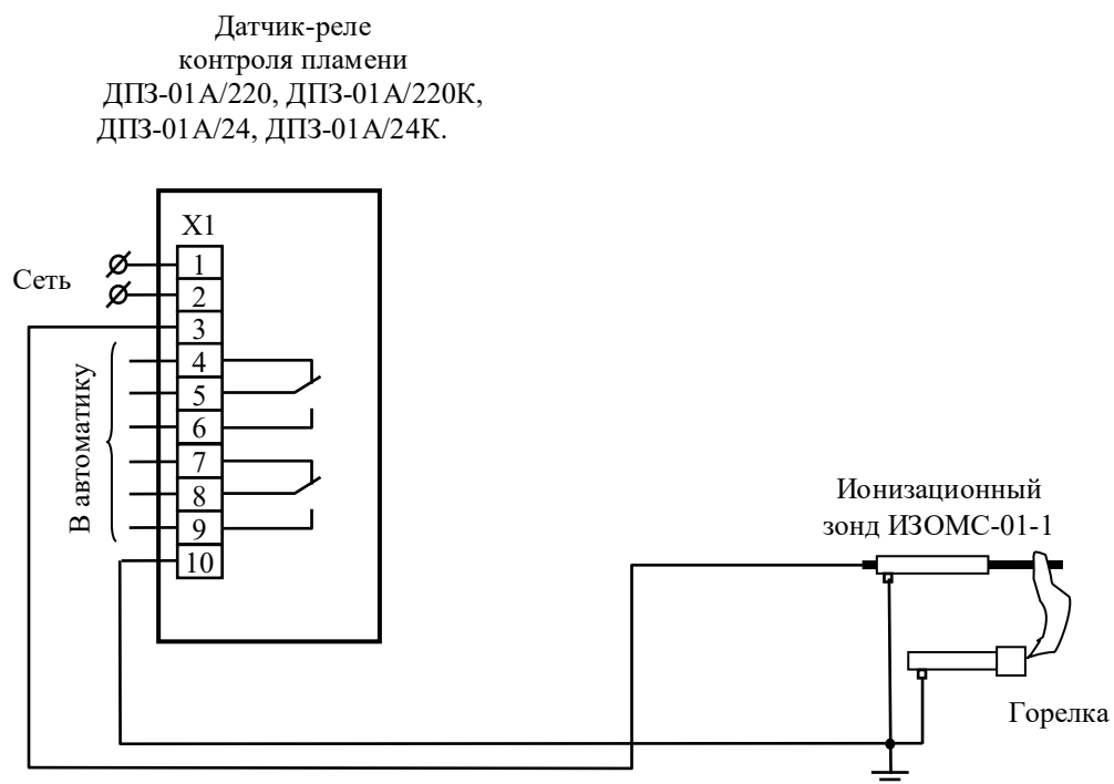
Рис. 2. Схема подключения датчика-реле контроля пламени ДПЗ-01А.
