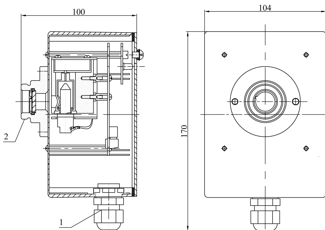
Рис. 1б. Общий вид датчиков реле контроля пламени ПАРУС-002УФ-1/24ЕК и Парус-002УФ-1/220ЕК. 1 – клеммная колодка, 2 - посадочная резьба датчика (G 1").
