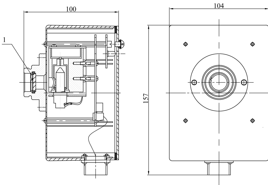
Рис. 1а. Общий вид датчиков реле контроля пламени ПАРУС-002УФ-1/24Е и Парус-002УФ-1/220Е. 1 – посадочная резьба датчика (G 1").
