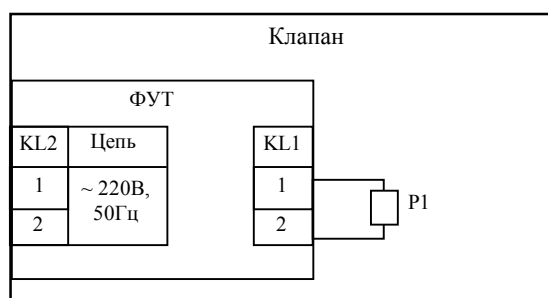
Рис. 3 Принципиальная электрическая схема клапана ЭМКГ8-15-40-220-с298-10. P1 – катушка; ФУТ – формирователь управляющего тока.
