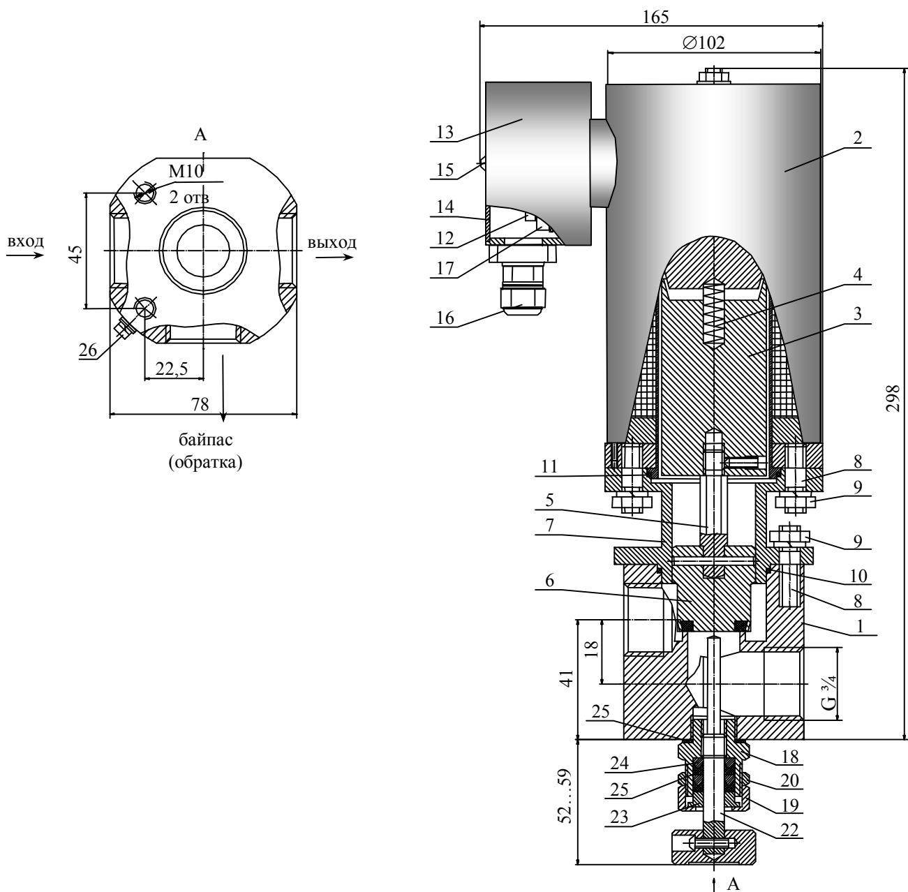
Рис. 2. Устройство клапана ЭМКГ8-20-25-220-с324-10.
