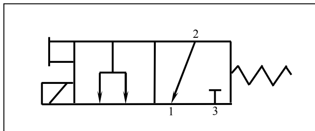
Рис. 1. Функциональная схема клапана. 1 – рециркуляция; 2 – вход клапана; 3 – выход клапана.
